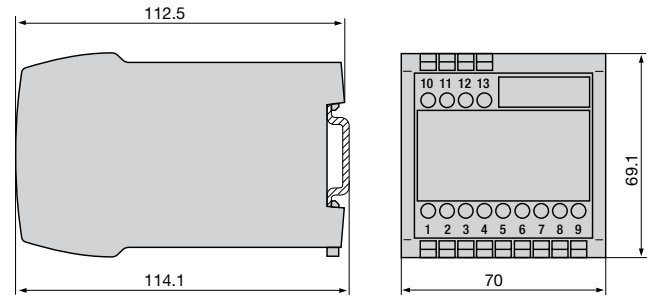
Fig. 7. Boîtier type P13/70 encliqueté sur rail «à chapeau» (35 x 15 mm ou 35x7,5 mm, selon EN 50 022).
