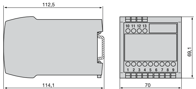
Bild 7. Gehäuse P13/70 auf Hutschiene (35 x 15 mm oder 35 x 7,5 mm, nach EN 50 022) aufgeschraubt.
