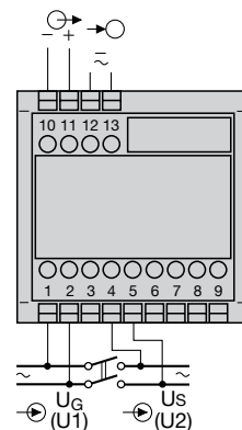
Fig. 4. Alimentation auxiliaire sur côté basse tension sur bornes 12 et 13.
