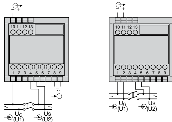
Bild 3. Hilfsenergie intern ab Messeingang, Hilfsenergie-Anschluss entfällt.
